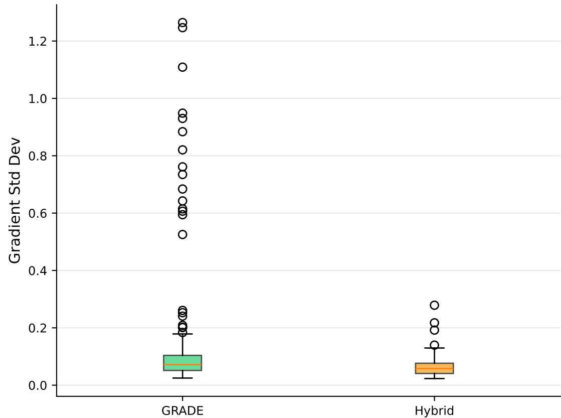
(b) Gradient Variance
